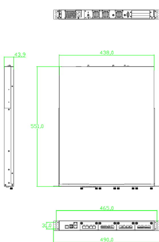
a. ATL-C236N4-RP
