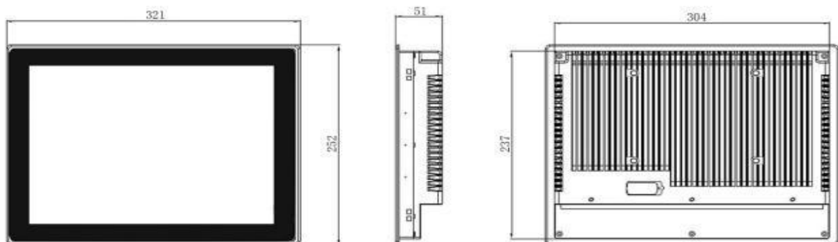
开孔尺寸: 306x239mm
